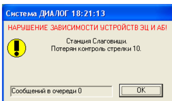
Рис. 8. Предупреждение «Нарушение зависимости устройств ЭЦ и АБ!».
