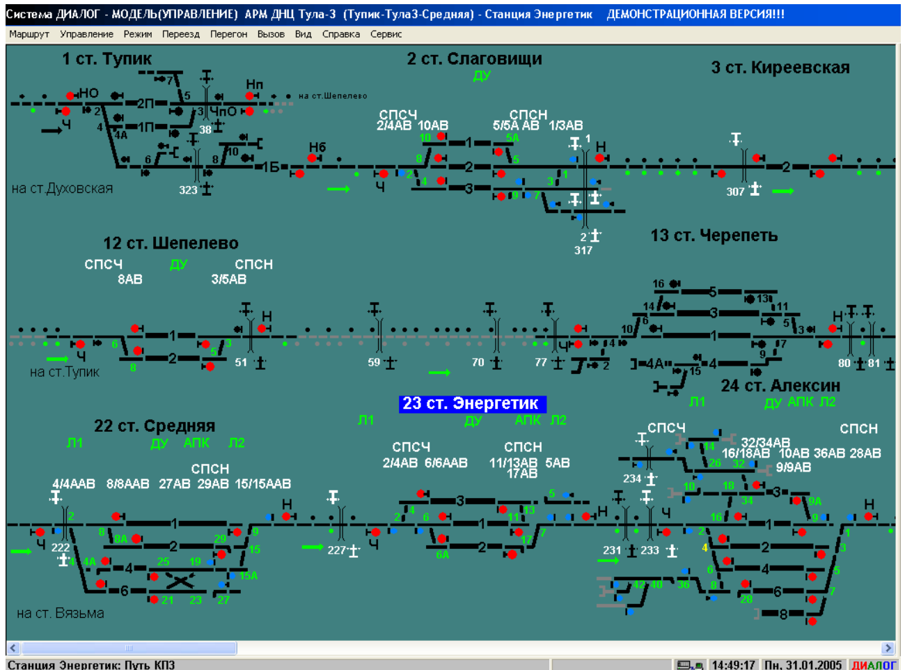
Рис. 1. Пример отображения основного экрана АРМ УДП.
